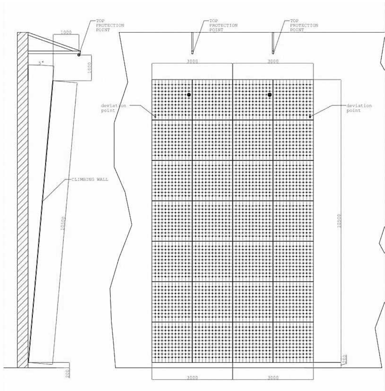
図 8.2 ( a ) 10m 競技用レーン
